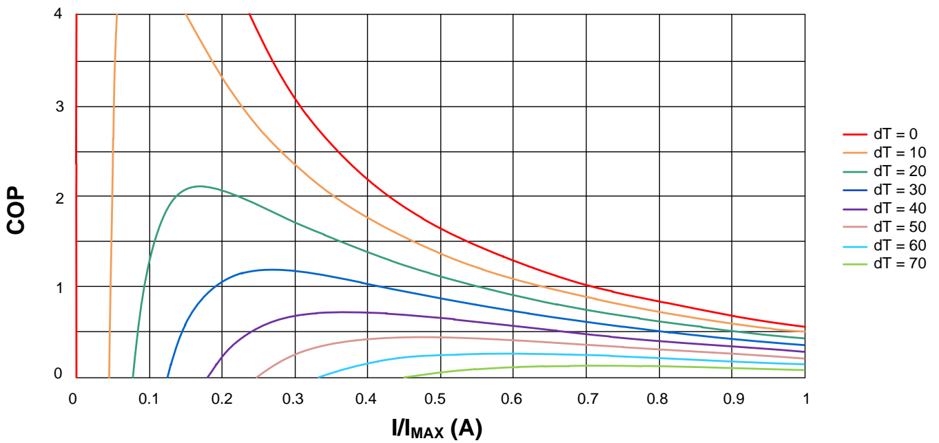
图 11. COP vs. I/I_{MAX}
