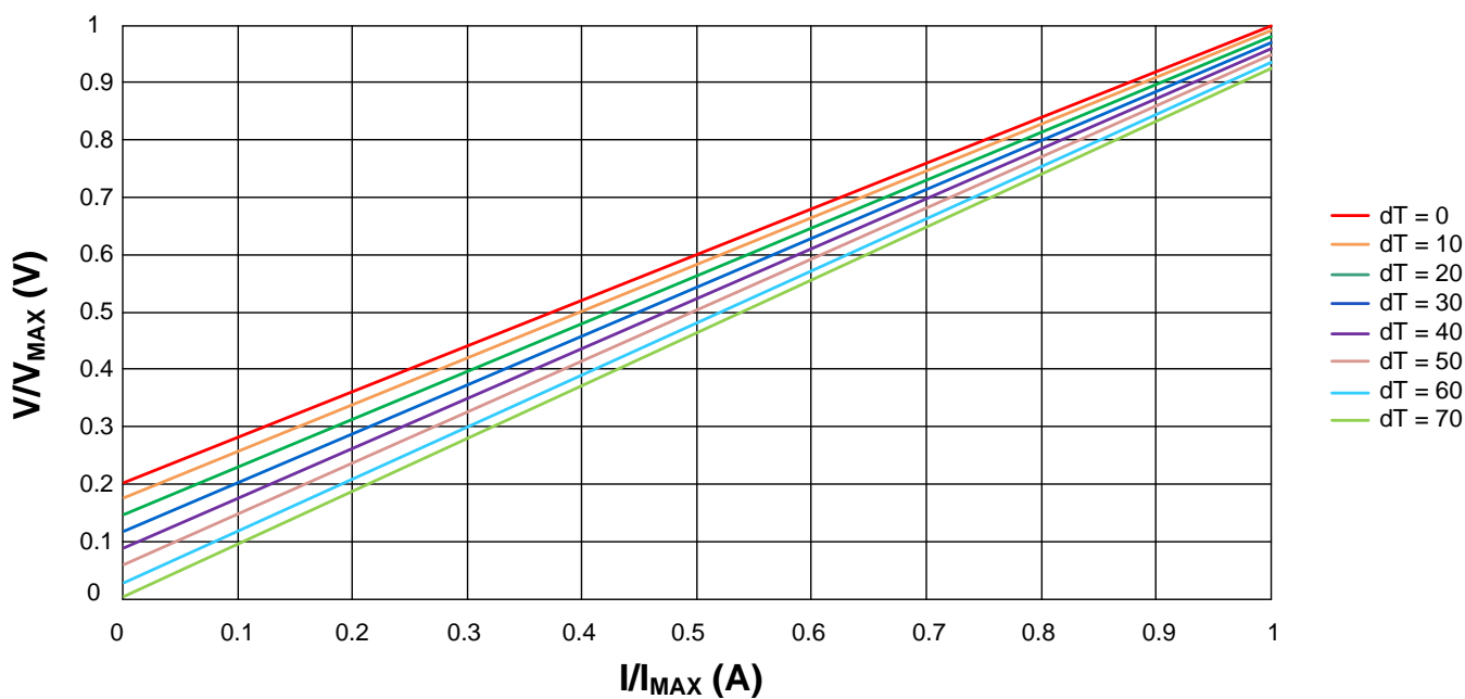
图 9. V/V_{MAX} vs. I/I_{MAX}
