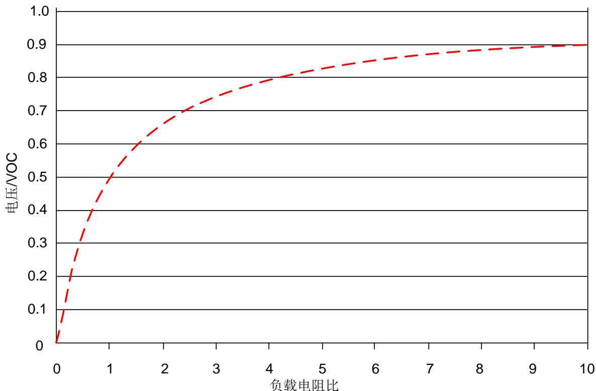
图 20. 负载电阻比 vs. 电压/VOC
