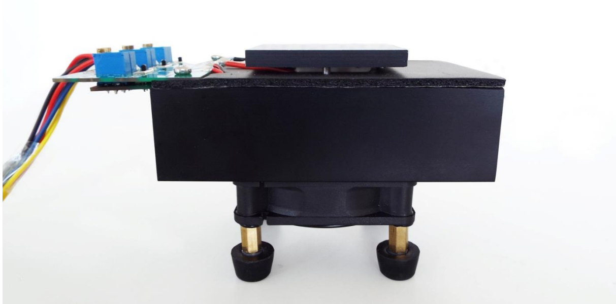
图 7. 侧视图
