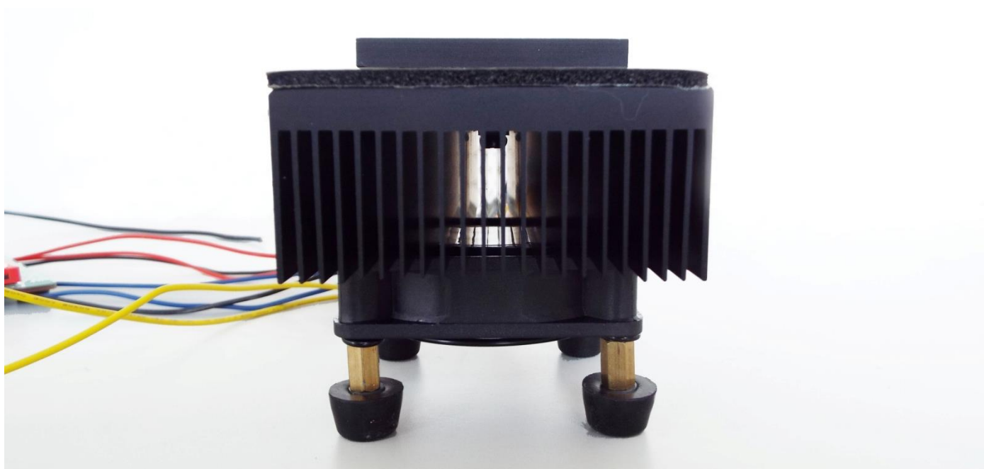
图 8. 侧视图
