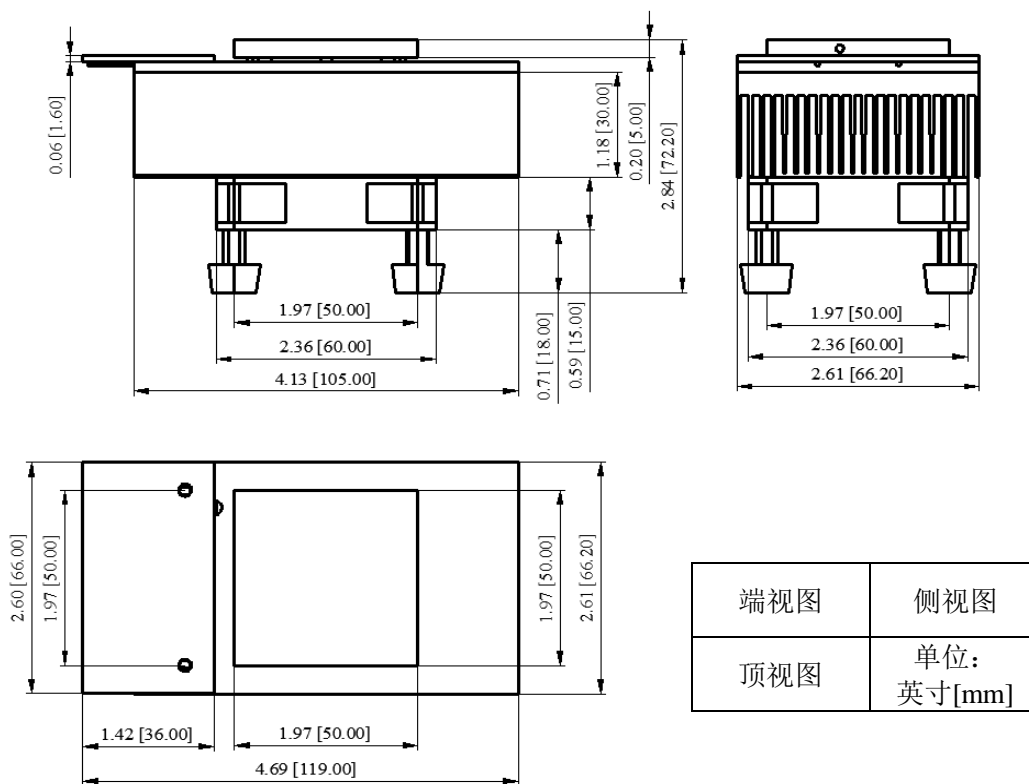
图 10. ATTP1A 尺寸图
