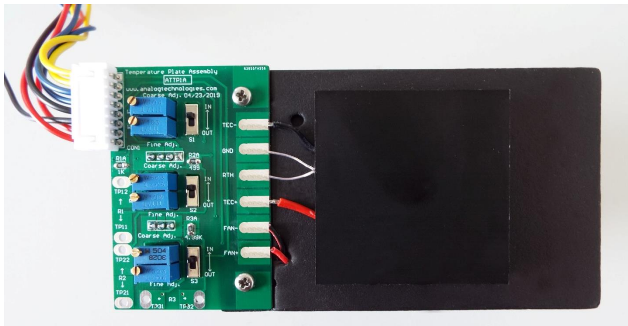
图 2. ATTP1A 实物图片
