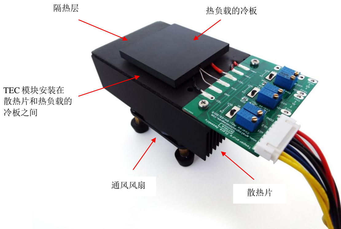
图 9. 图解说明
