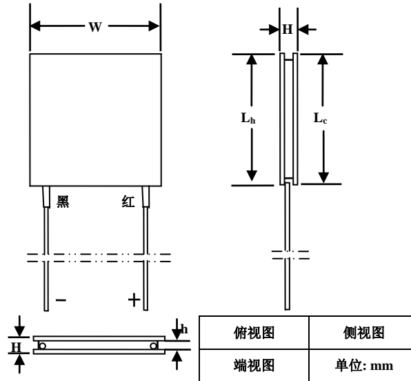
图2. ATE1-TC-71的机械尺寸
